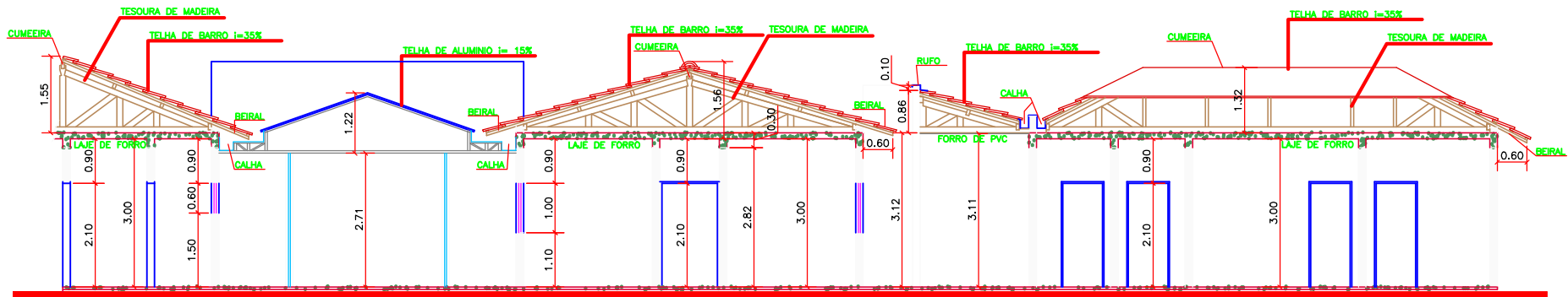
CORTE BB ESCALA = 1:50
