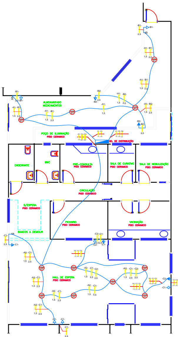
PROJETO ELÉTRICO Esc. 1:100
