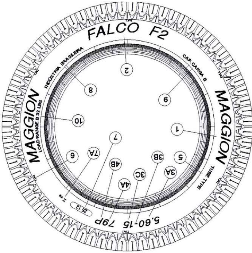
INFORMAÇÕES TÉCNICAS NA LATERAL DO PNEU
