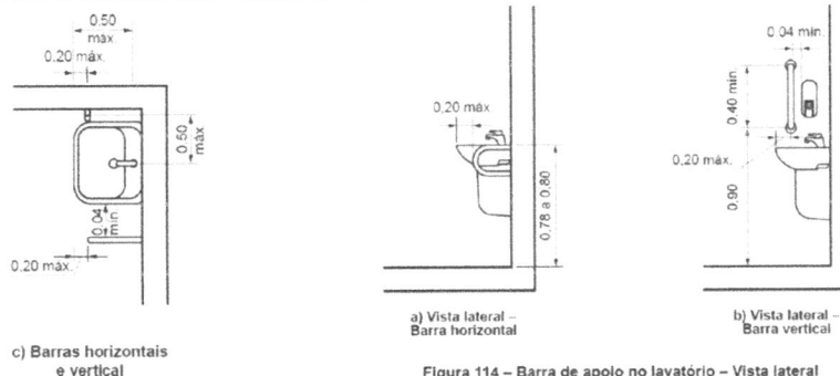
Figura 114 – Barra de apoio no lavatório – Vista lateral
