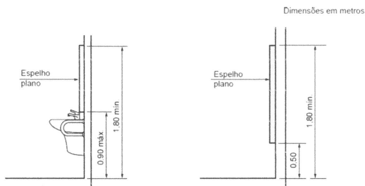
Figura 122 – Altura de instalação do espelho – Vista lateral
