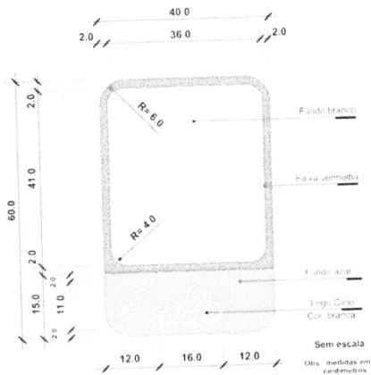
Padrão de placa de advertência para ciclovia:
