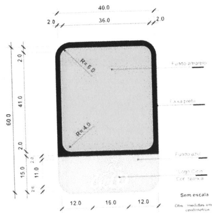
Placas de regulamentação:
