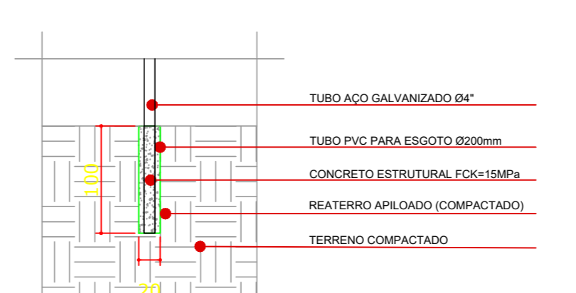
FUNDAÇÃO TRAVE sem escala
