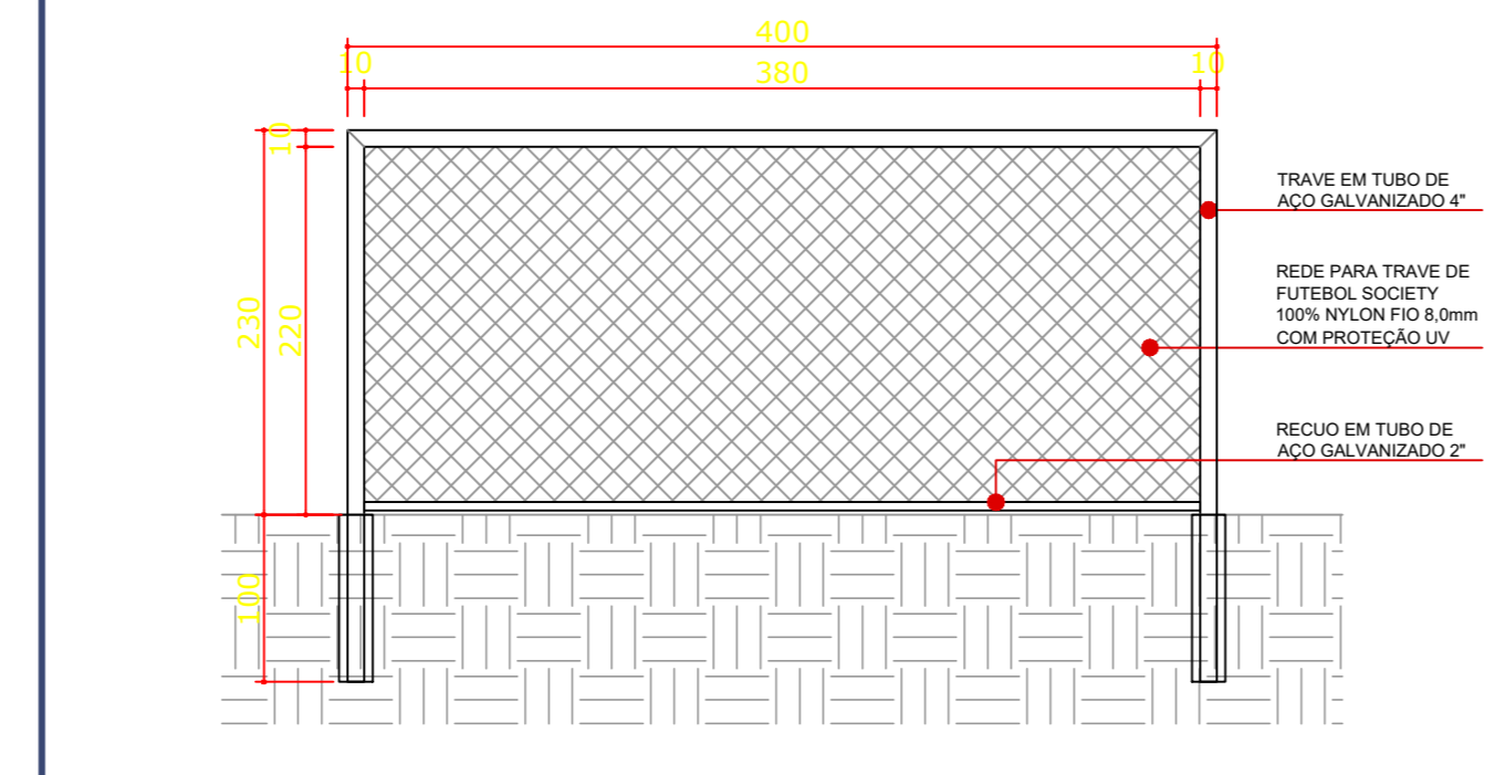
VISTA TRAVE sem escala
