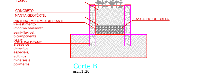
Corte B esc: 1:20
