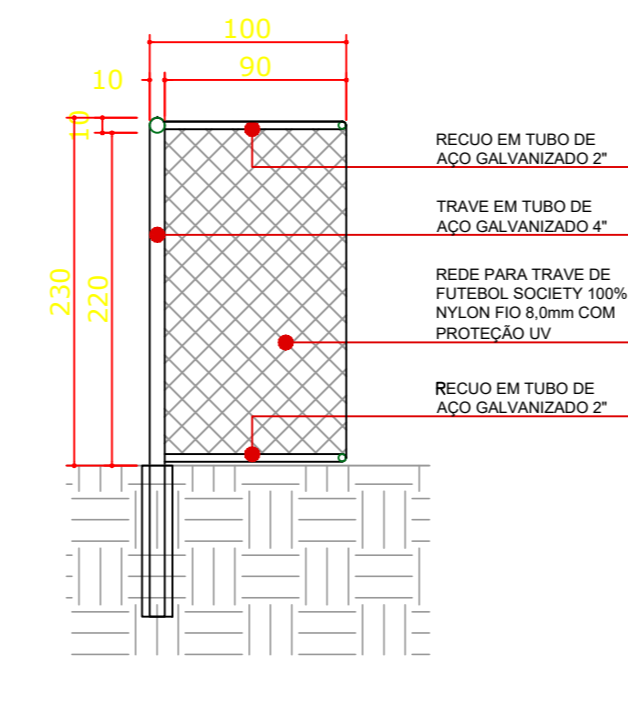
CORTE TRAVE sem escala
