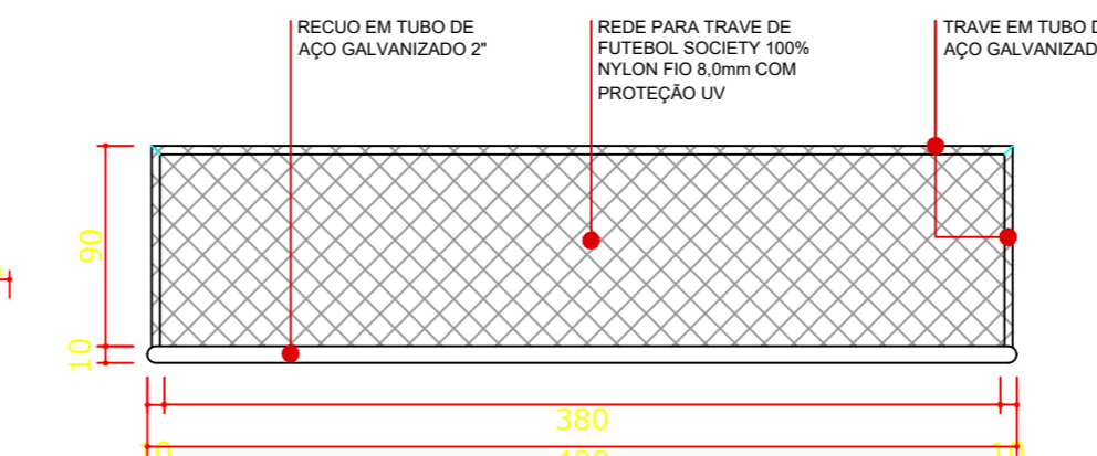
PLANTA TRAVE sem escala
